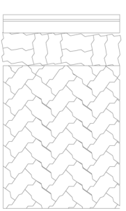
04 | DET. PASSEIO esc.: 1:25
