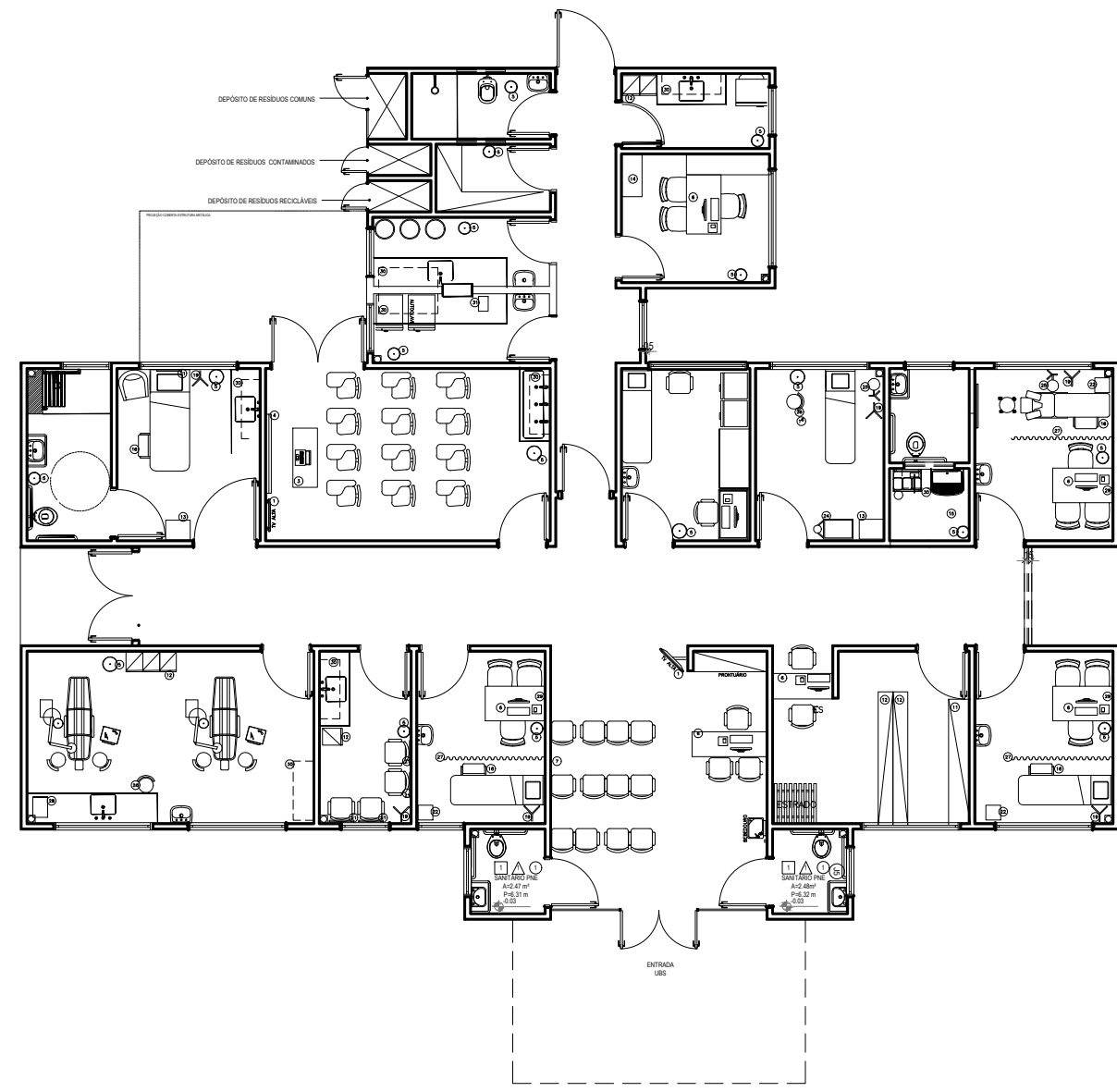
1 PLANTA DE LAYOUT ESCALA 1:50
