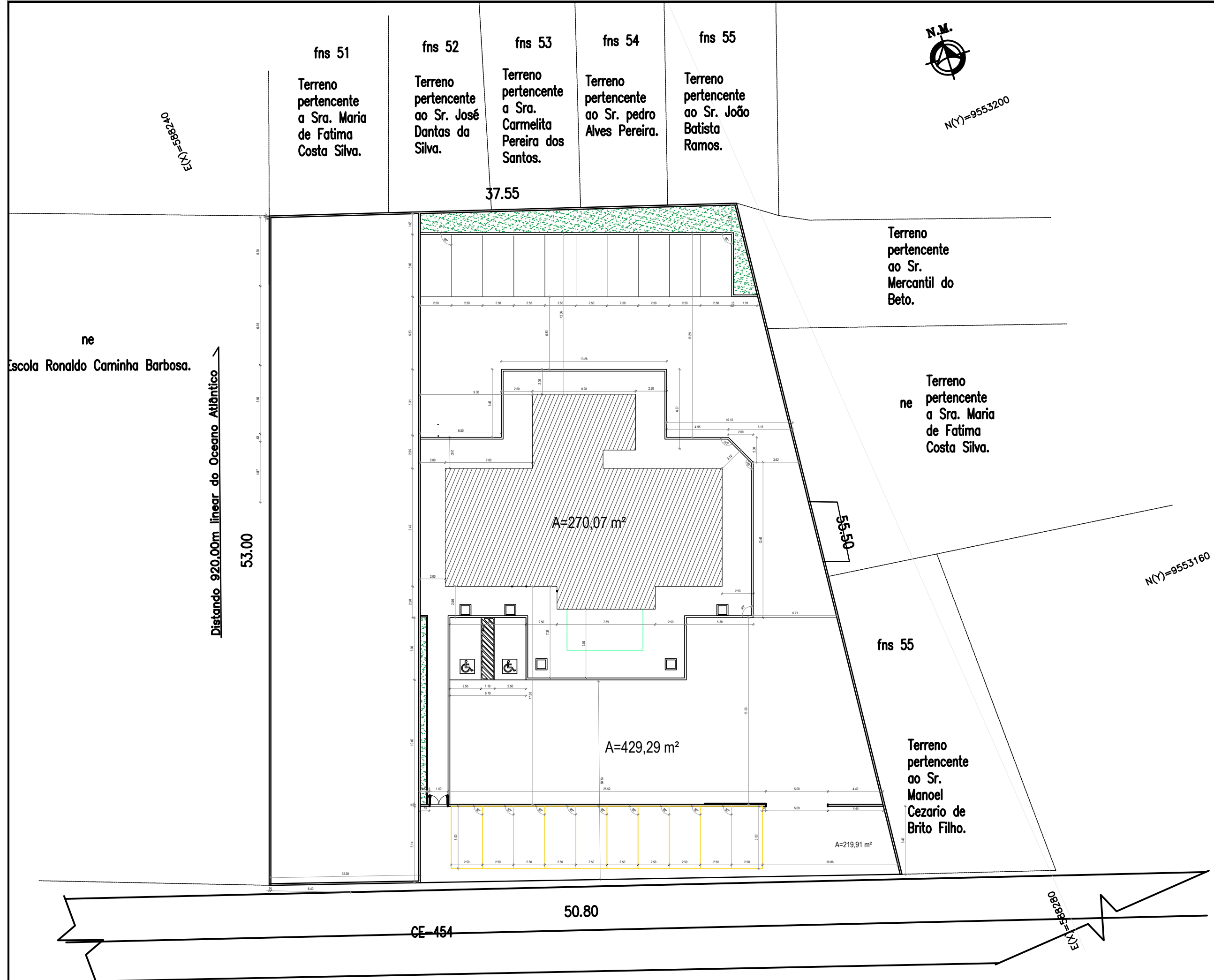
1 SITUAÇÃO E LOCAÇÃO ESCALA: 1:100
