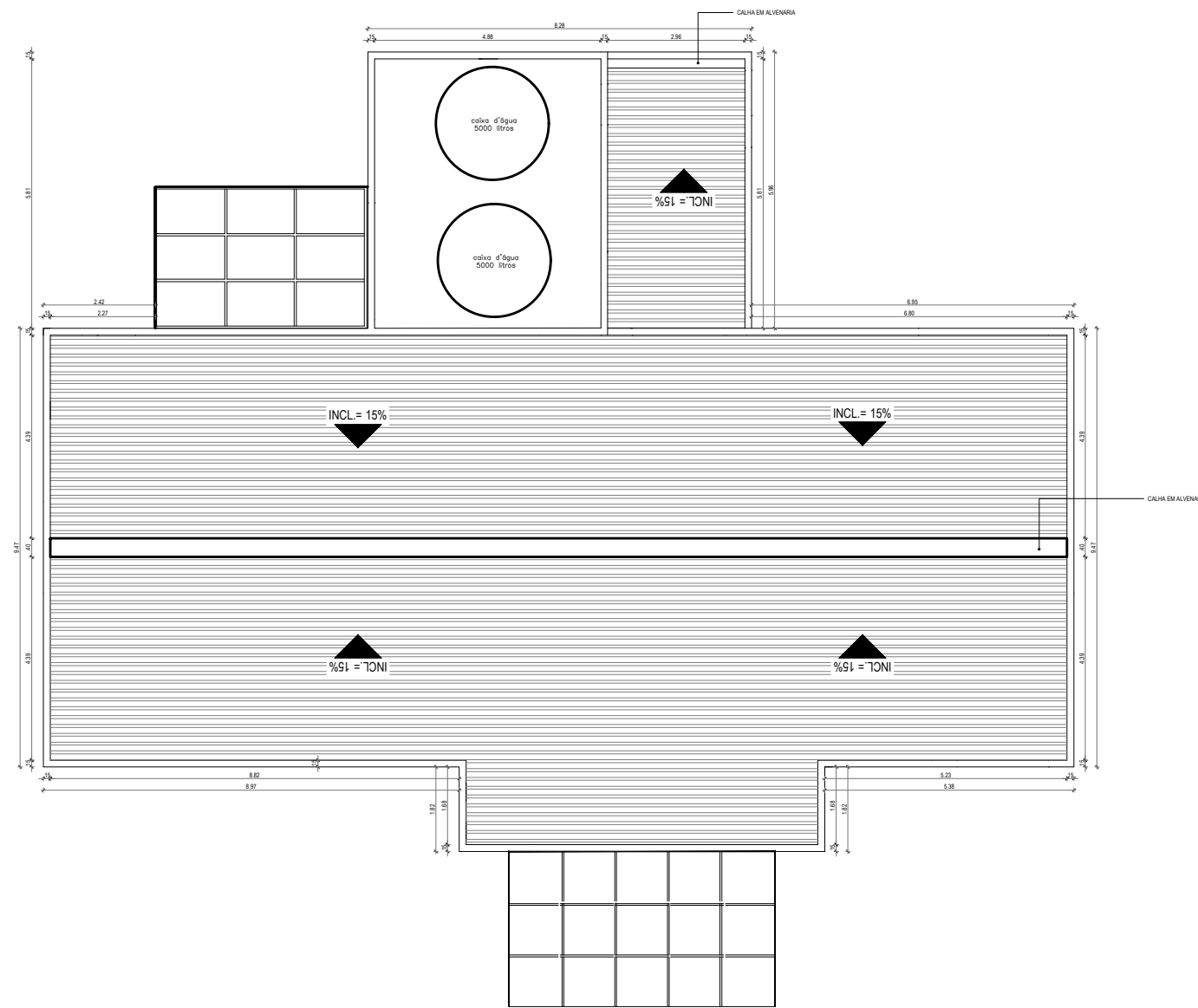
1 PLANTA DE COBERTA ESCALA 1:50
