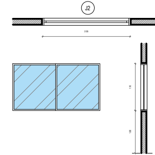
04 DET. ESQUADRIA J2
