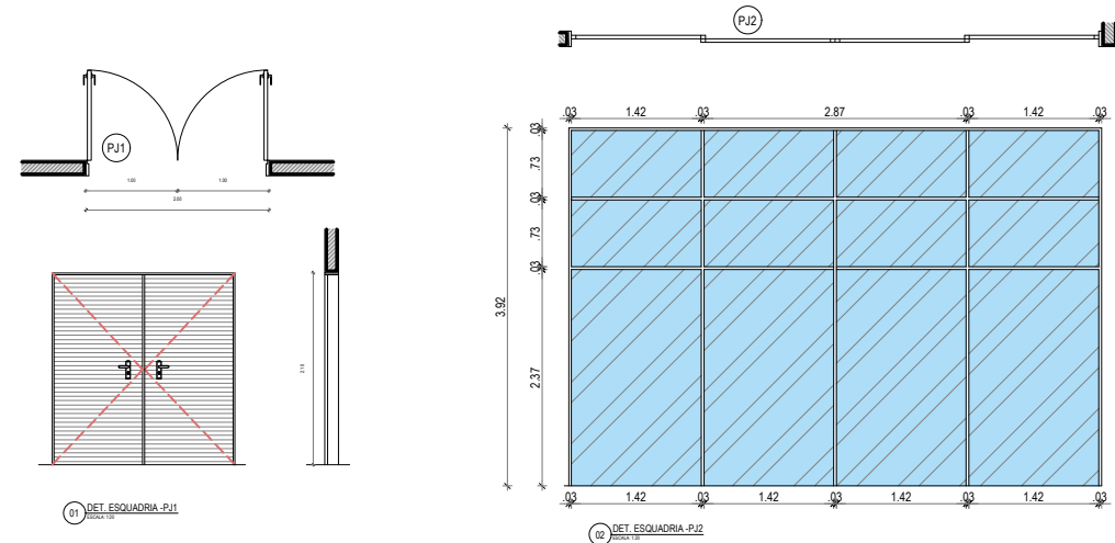
02 DET. ESQUADRIA P12
