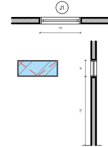
03 DET. ESQUADRIA J1
