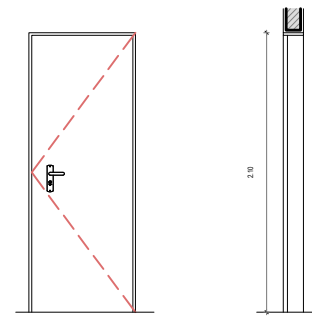
03 DET. ESQUADRIA - P3 ESCALA 1:20
