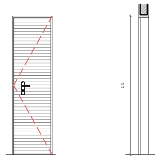
05 DET. ESQUADRIA - P5 ESCALA 1:20
