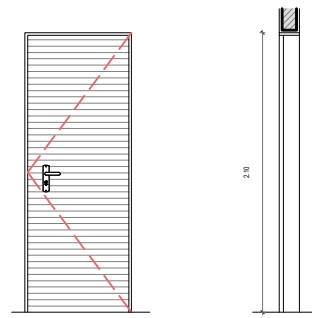
01 DET. ESQUADRIA - P1 ESCALA 1:20
