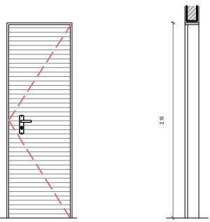
02 DET. ESQUADRIA - P2 ESCALA 1:20
