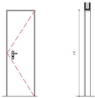
04 DET. ESQUADRIA - P4 ESCALA 1:20
