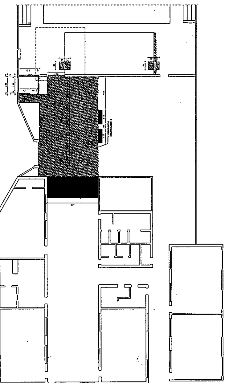
01 PLANTA DE REFORMA - RAMPA
